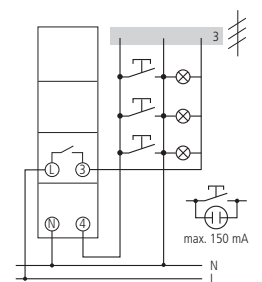
ELPA 6, ELPA 6 plus, ELPA 7
