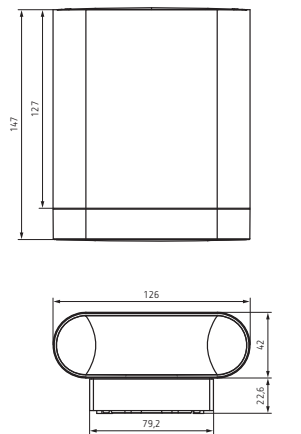
theLeda D U AL
