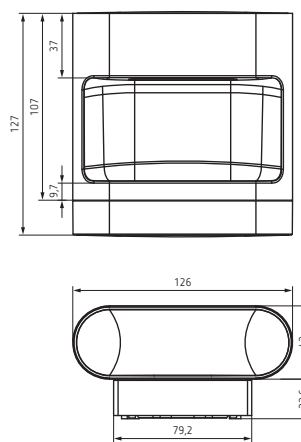
theLeda D S AL
