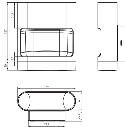
theLeda D SUL AL
