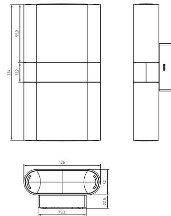
theLeda D UD AL
